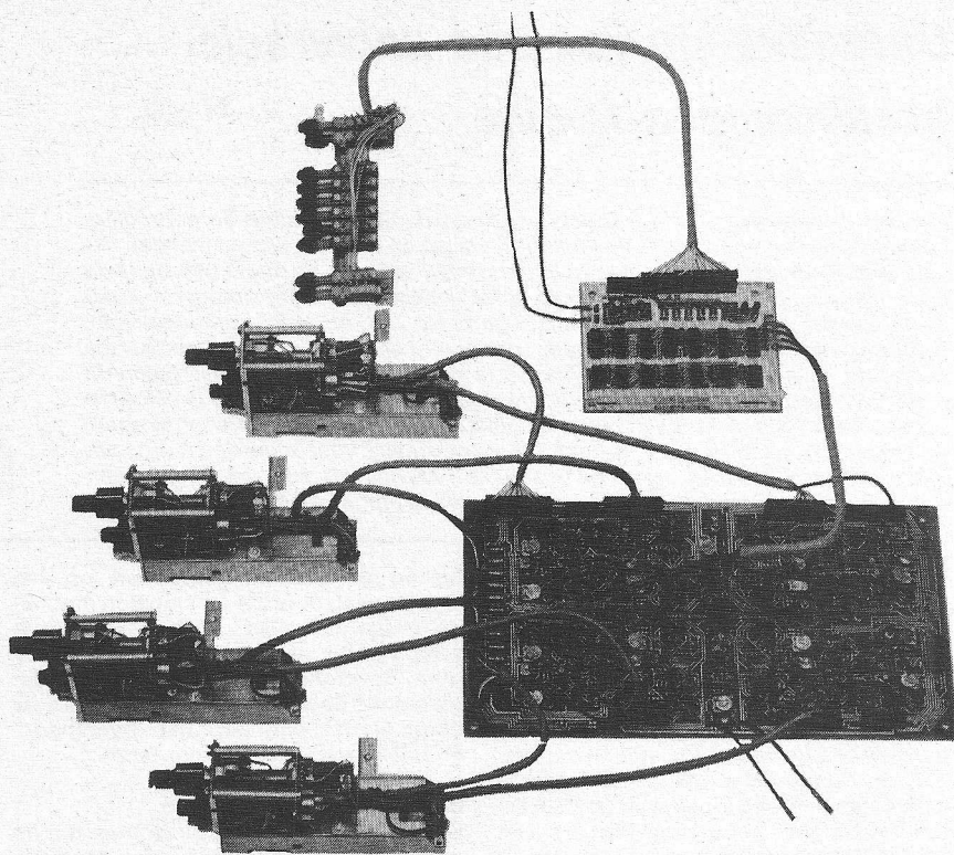
Afb. 2. Enkele gescheiden functionele eenheden van de PM 3244. Linksboven de beeldkeuze-instelling, via een kabelboom verbonden met de beeldkeuze-logica. De commando's worden met een viertal gebundelde coax-kabeltjes overgebracht naar de grote printkaart, waarop zich de verticale omschakelpoorten bevinden. Tevens zijn hier de symmetrisch opgebouwde verticale ingang-versterkers ondergebracht. Elke sectie is door een dubbele kabelbundel verbonden met de verzwakker/voorversterker ingangsmodule. Door deze „koude“ schakeltechniek is het aantal mechanische componenten drastisch verminderd.
