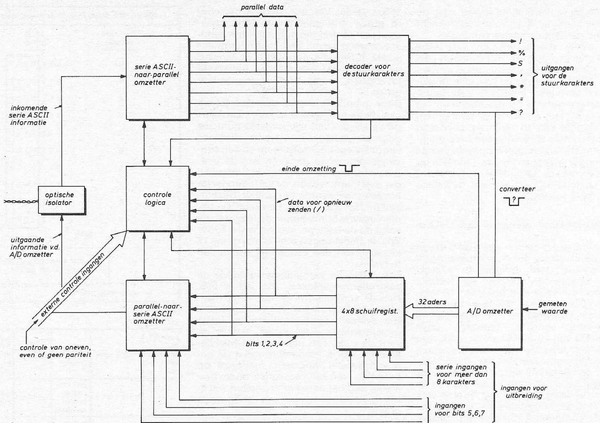
Fig. 3. Serie-zender.
