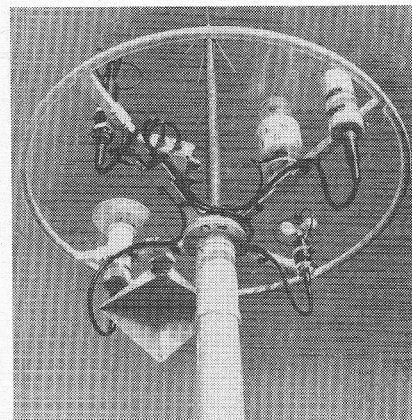
Masttop van de L55/Nimbus 6 boei, waarin de verschillende sensoren en de UHF-antenne zijn verwerkt.
