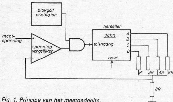
Fig. 1. Principe van het meetgedeelte.
