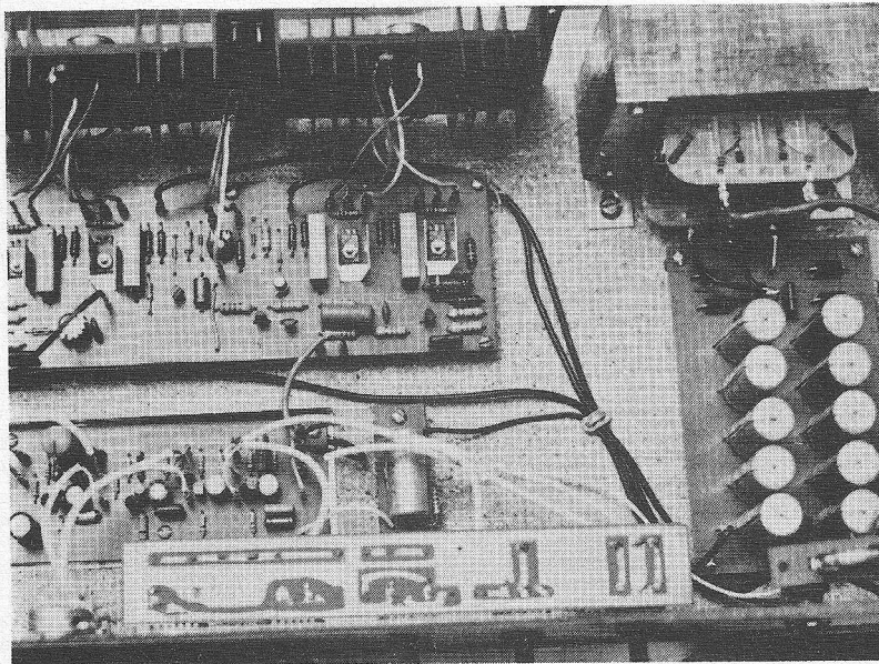
Eindversterker als onderdeel van een gitaarversterker.
