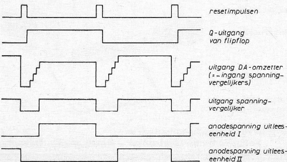
Fig. 4. Enkele optredende spanningvormen op diverse punten.
