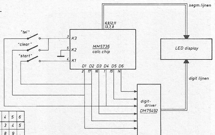
Fig. 3. Eenvoudige 6-decaden teller.
