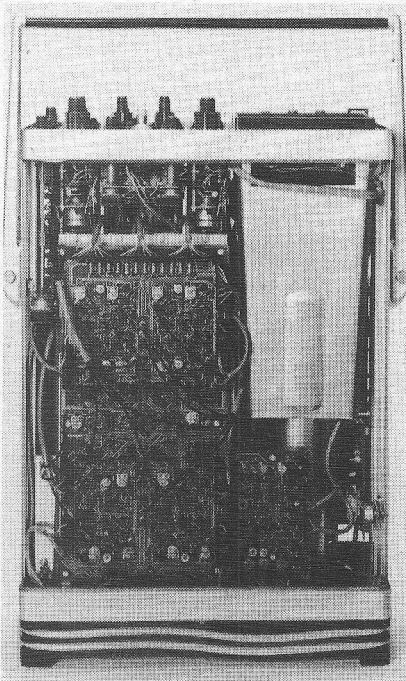
Afb. 3. Boven-aanzicht van de geopende PM 3244. De complete elektronica van de voorgaande afb. is keurig opgeborgen naast de beeldbuis. Let op de compacte, maar ontegenzeggelijk service-vriendelijke opbouw.
