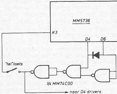
Fig. 7. Schakeling voor het verhogen van de telfrequentie.
