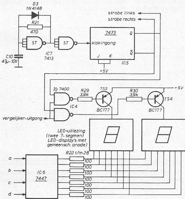
Fig. 3b. Sturing en omschakeling van decoder-indicatoren.
