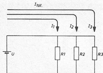
Fig. 60: Bij parallel geschakelde weerstanden is de totale stroom gelijk aan de som van de deelstromen.
