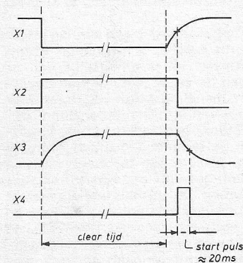
Fig. 5. Tijdrelatie tussen „clear” en „start”.
